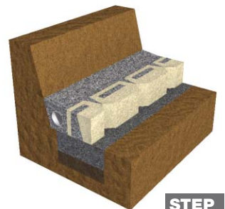
STEP
